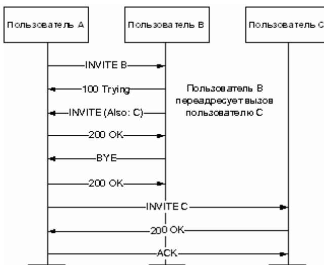
Рис. 12 Дополнительная услуга "Переадресация вызова"
