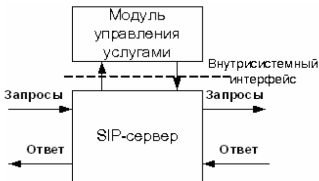
Рис. 4 Структурная схема организации услуг SIP-сервера
