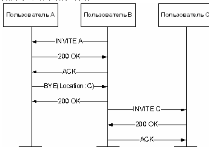
Рис. 11 Дополнительная услуга "Переключение связи"
