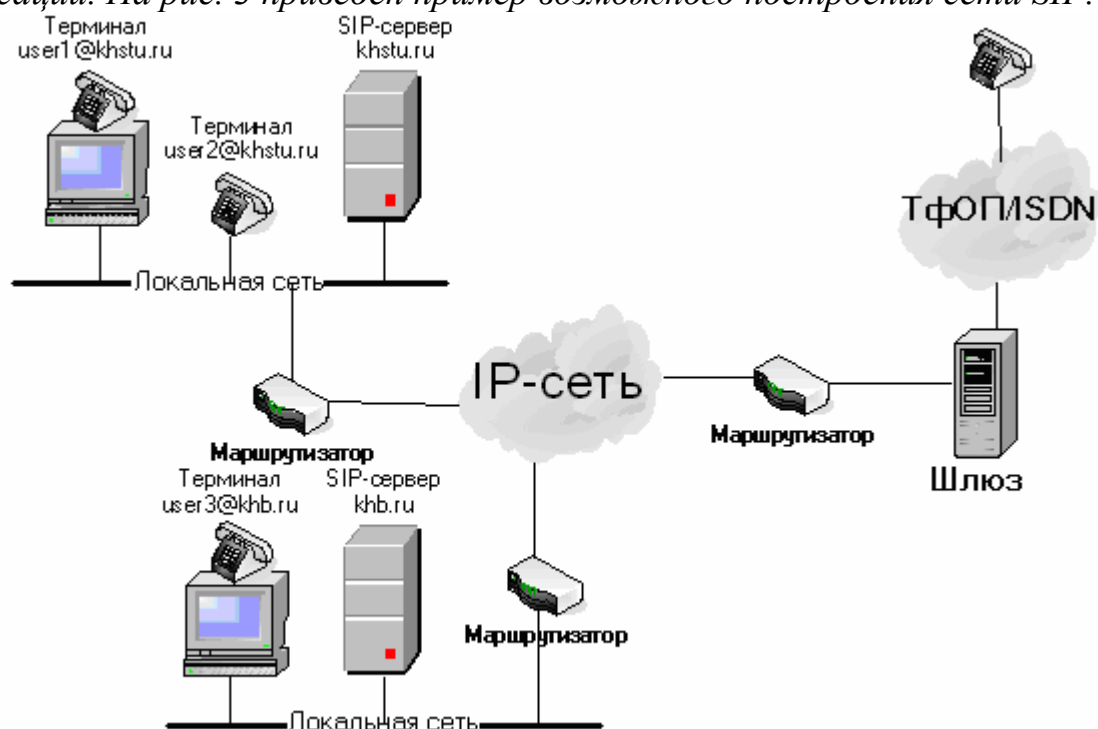
Рис. 3 Пример построения сети SIP
