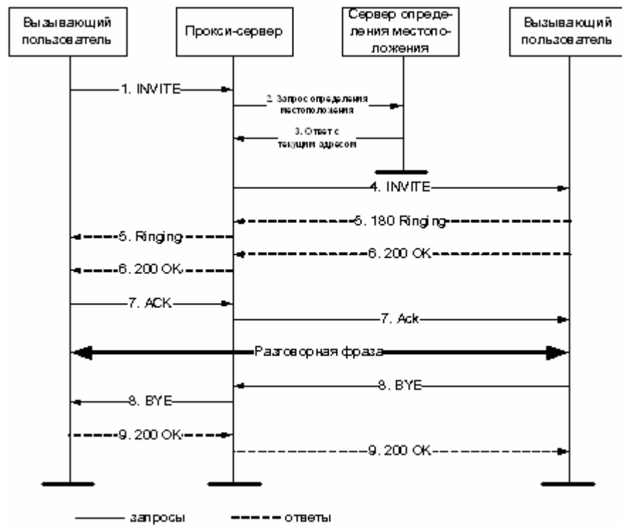
Рис. 10 Сценарий установления соединения через прокси-сервер
