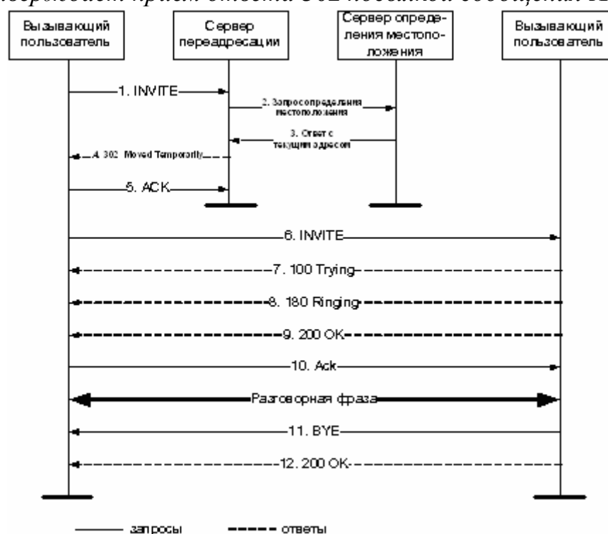
Рис. 9 Сценарий установления соединения через сервер переадресации
