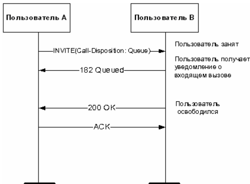
Рис. 13 Дополнительная услуга "Уведомление о вызове во время связи"
